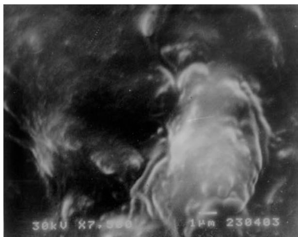
Slika 2. SEM mikrograf NR/CSM/ERP kompozita sa dodatkom 20 phr recikliranog gumenog praha pri uvećanju od 7500 puta
